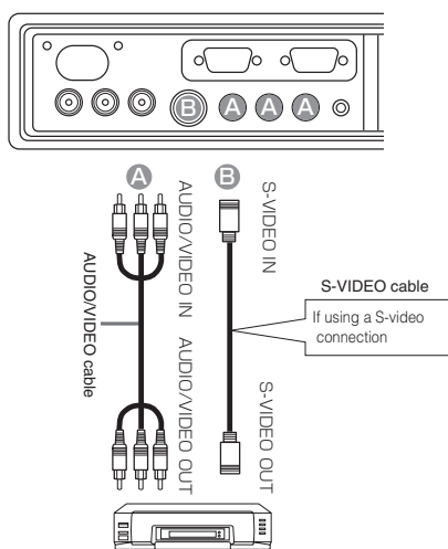
VCR
