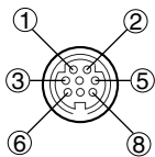
DIN 8 clavijas Aspecto exterior
